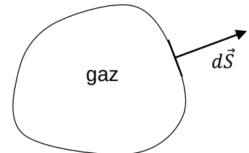
Gaz contenu dans un récipient. Élément de surface de la paroi
