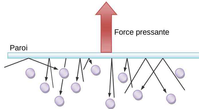
Document 5 – Le choc des molécules contre une paroi provoque une force pressante
