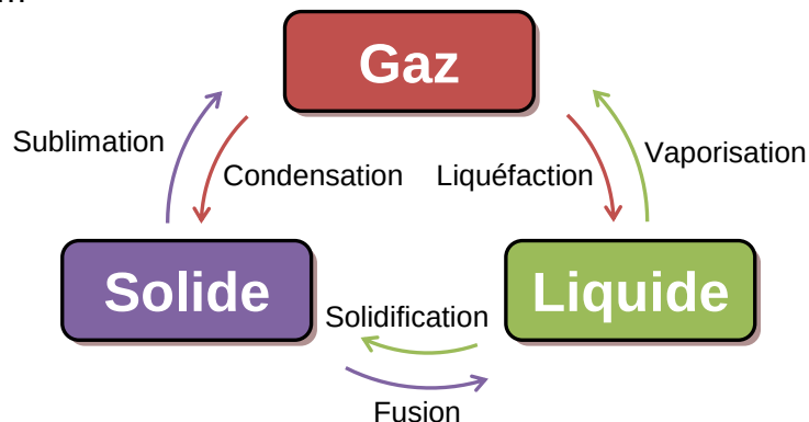
Document 10 – Les différents changements d'état de la matière
