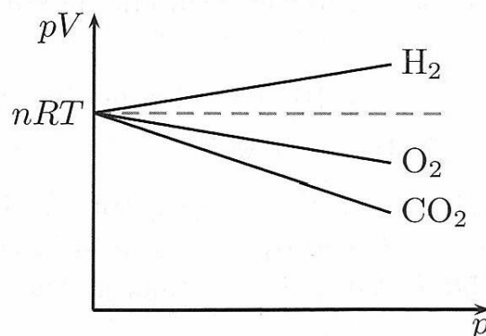
Document 9 – Diagramme d'Amagat de gaz réels à basses pression et à 273 K, le modèle du gaz parfait est en pointillé.
