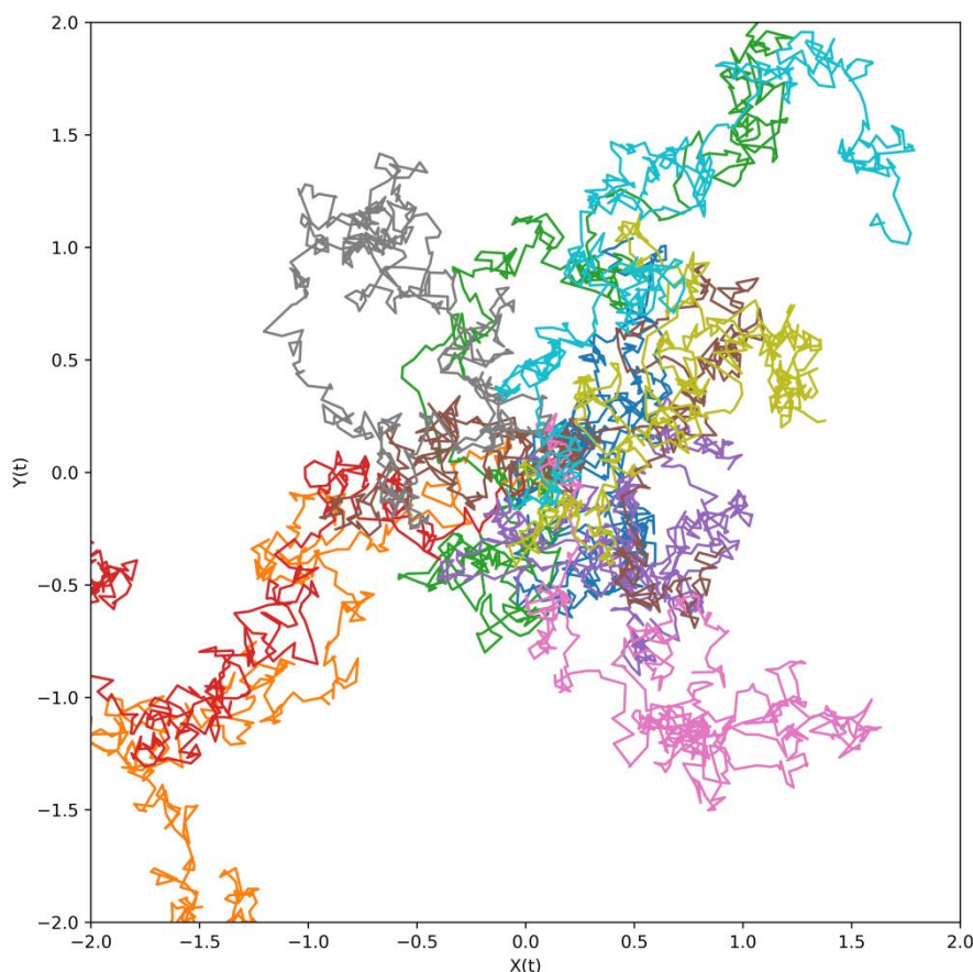
Document 2 – Simulation de 10 trajectoires browniennes.
